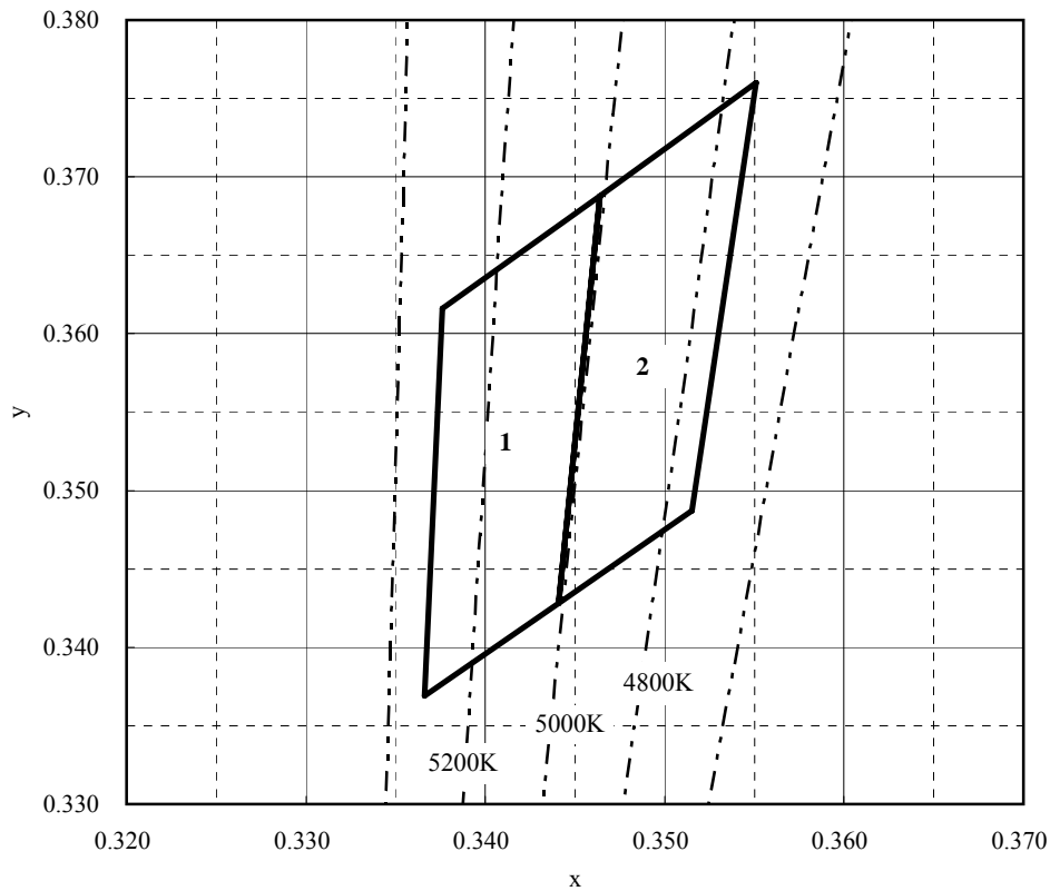
色度座標図
